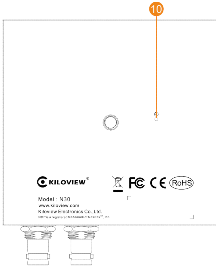
10.Reset button
